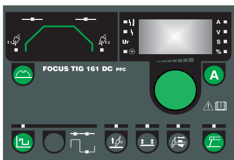
Betjeningspanel til Focus TIG 161 DC HP PFC
